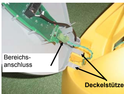
Abbildung 1.20 Zusammenbau der Basis und Deckel
