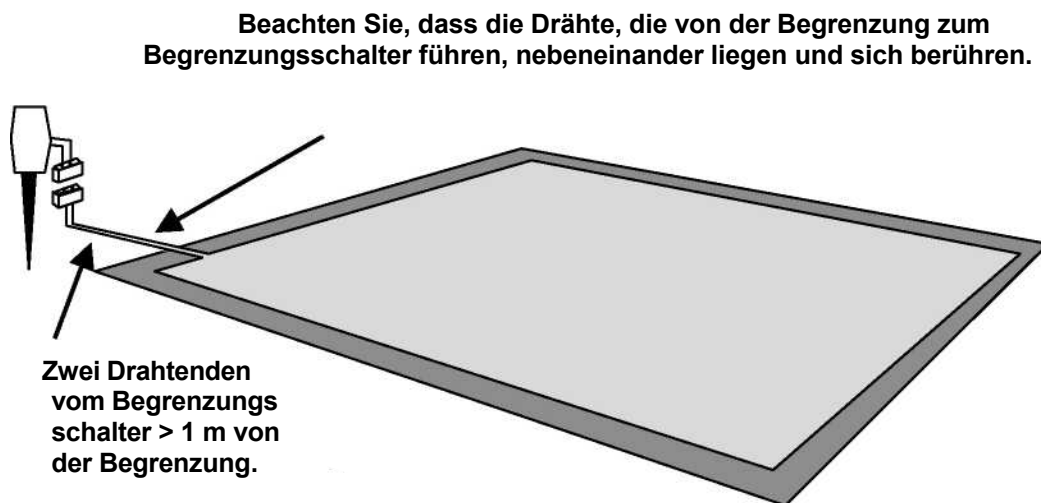
Abbildung 1.29 - Beendigung der Einrichtung beim Begrenzungsschalter
