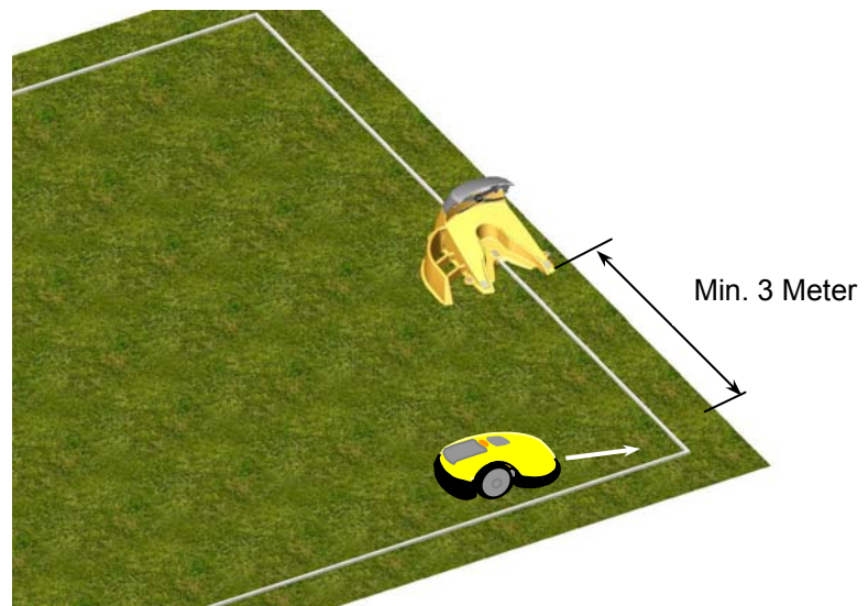
Abbildung 2.11 – Testen der Installation der Ladestation
