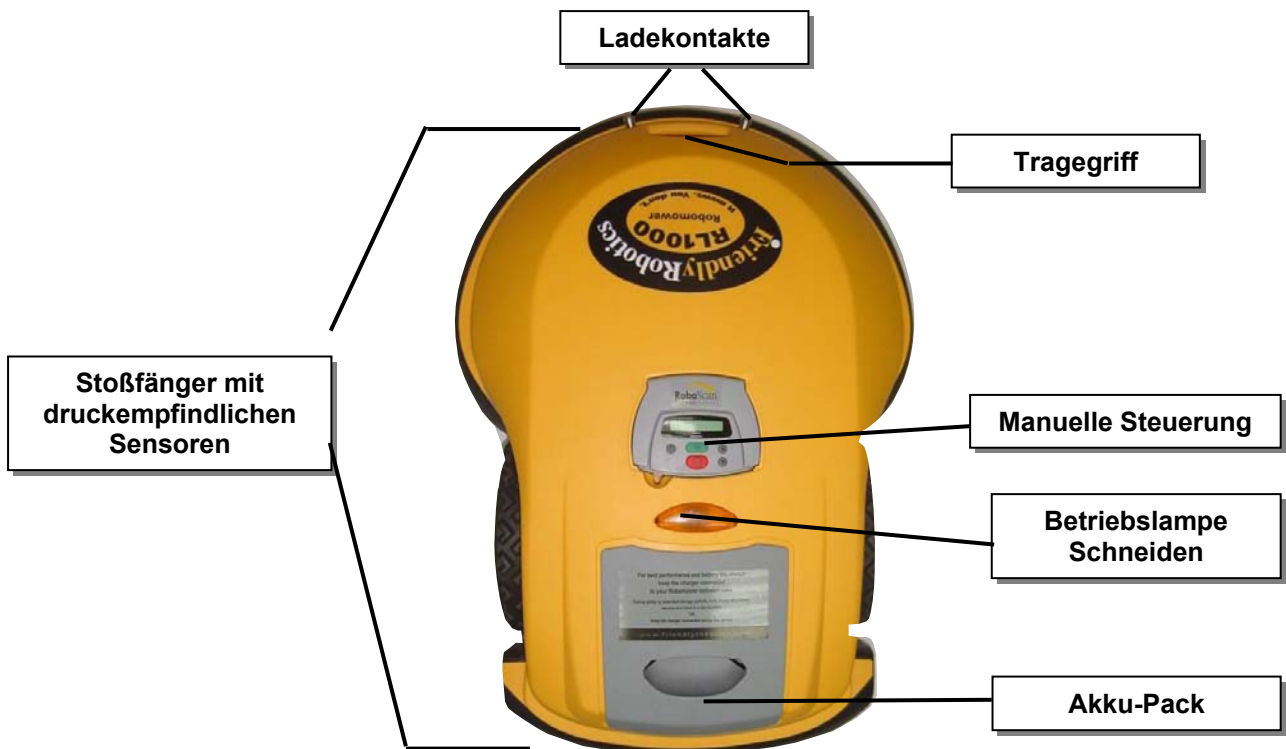
Abbildung 2.1 – Ein erstes “Was ist Was” beim Robomow®
