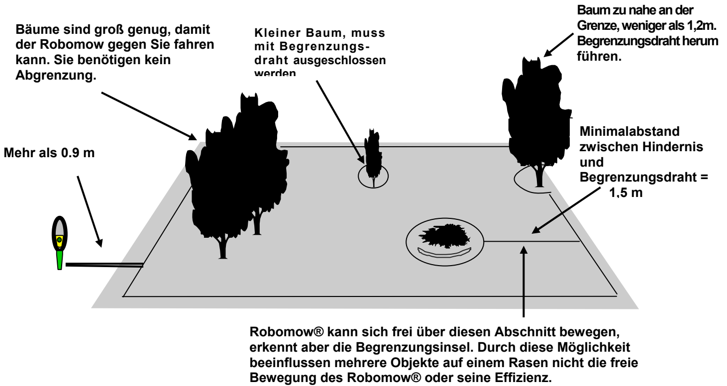
Abbildung 1.13 – Begrenzungsdraht installieren für Hindernisse
