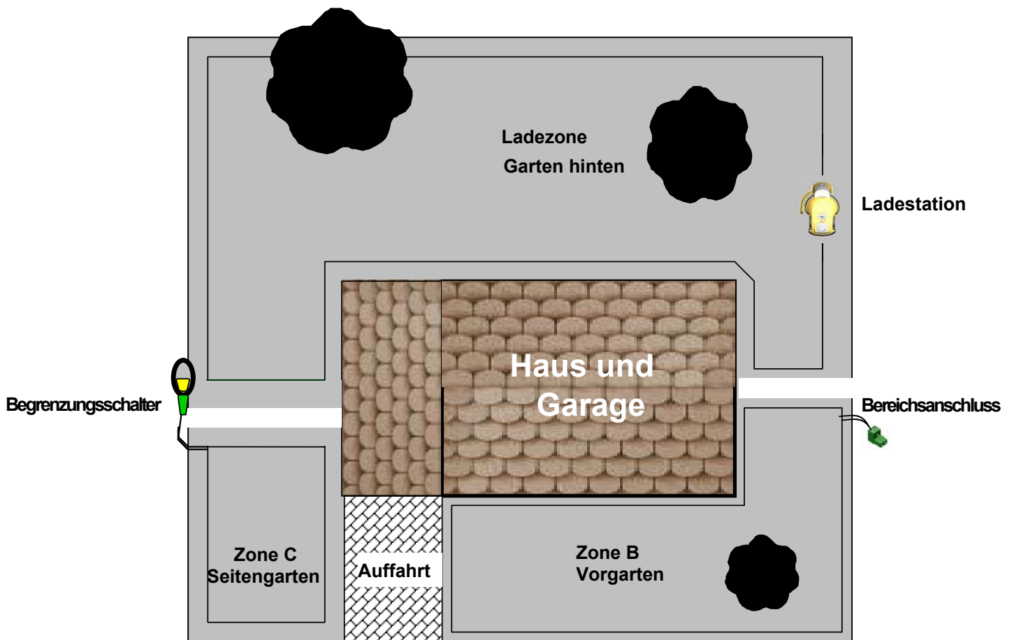
Abbildung 1.15 – Einen Begrenzungsschalter für mehrere Zonen
