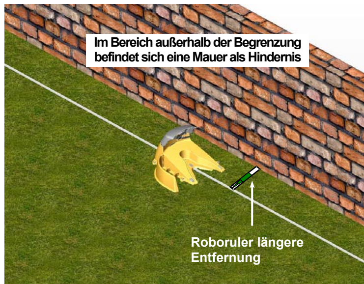
Abbildung 1.26 – Verwendung der längeren Entfernung des RoboRulers bei der Aufstellung der Ladestation
