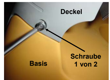
Abbildung 1.22 – Zusammenbau Basis und Deckel
