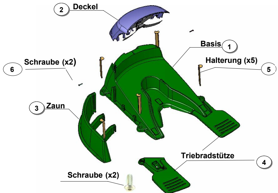
Abbildung 1.1 Ladestation komplett
