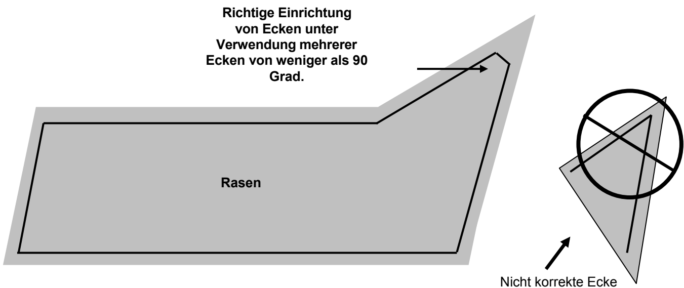
Abbildung 1.11 – Richtige Einrichtung bei scharfen Ecken
