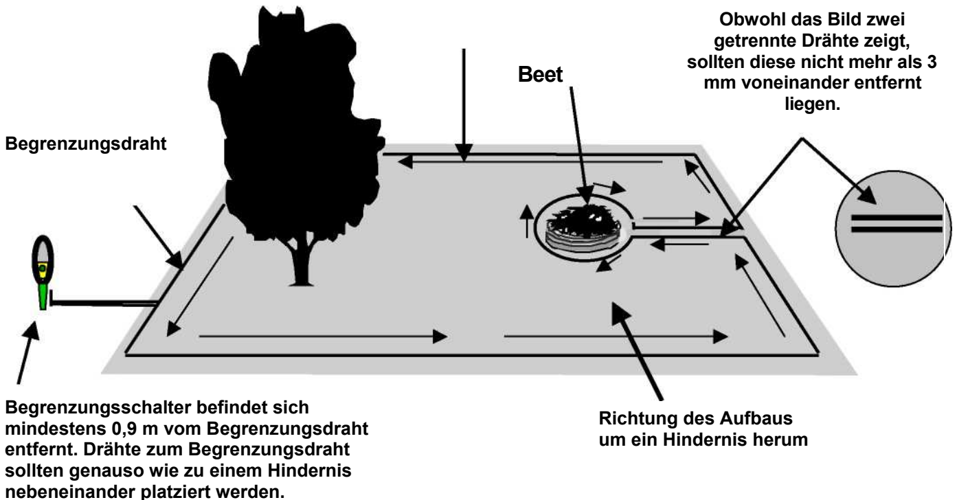
Abbildung 1.12 Objekte abschirmen mit dem Begrenzungsdraht
