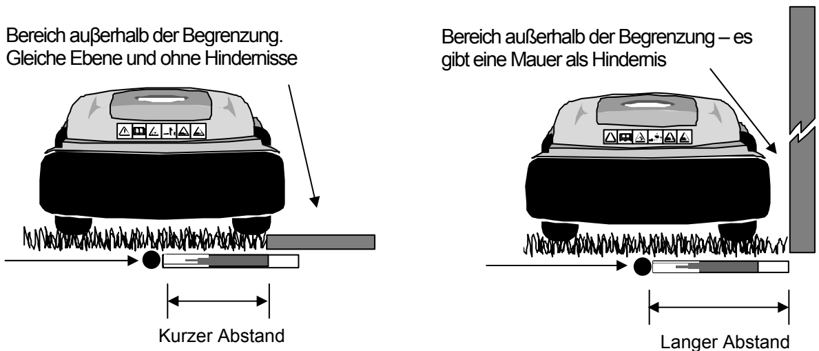
Abbildung 1.9 – Verwendung des RoboRulers
