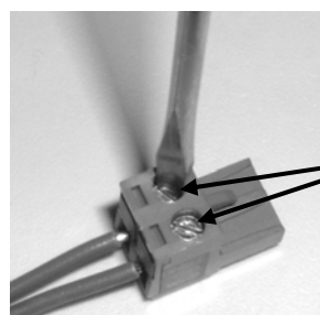
Abbildung 1.30 – Draht im Anschluss stecken und festschrauben
